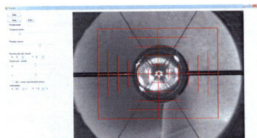
Рисунок 45. Система позиционирования измерительных антенн ГЭТ 158-2020
