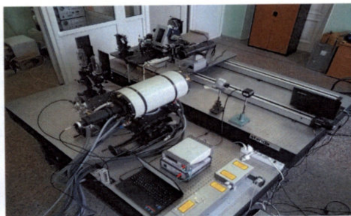
Рисунок 28. Установка из состава спектропрокомпаратора яркостей
